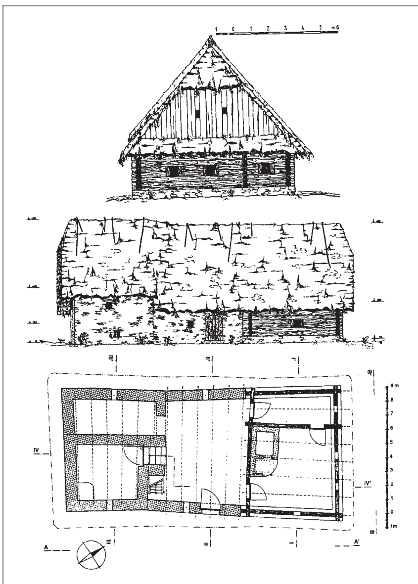
Obr. 10. Rekonstrukce a půdorys usedlosti ve středověké vsi Pfaffenschlag u Slavonic. Podle Vladimíra Nekudy. Kresba Zdeněk Špičák.
