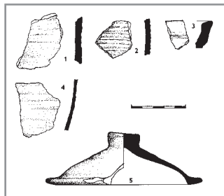
Obr. 26. Zlomky keramiky a zvoncovité poklice ze záchranného výzkumu v č. p. 51 (ul. Hlavní) v roce 1981. Kresba Rudolf Procházka.
